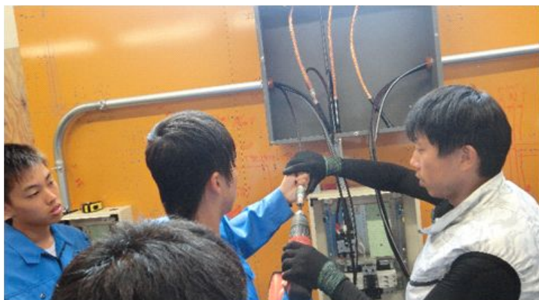
分電盤の幹線ケーブル接続作業
